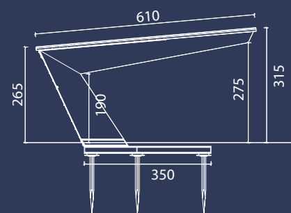
Seitenansicht FLASH
