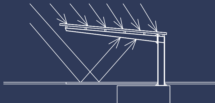
Wirkungsweise Bifacial Module
