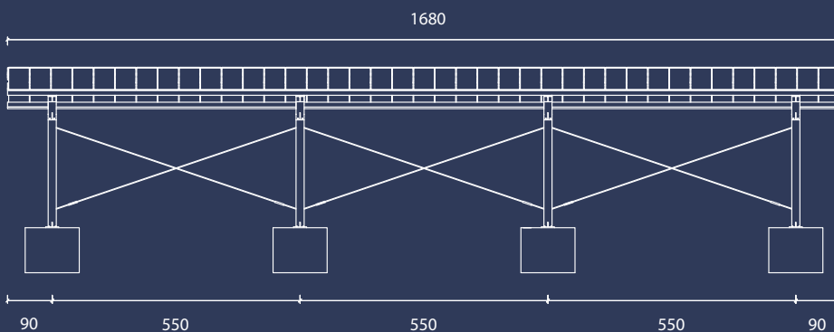
Frontansicht SUNSHELL
