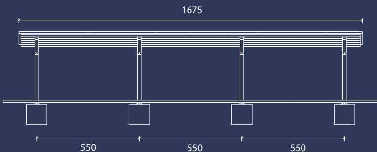
Frontansicht ESPACE
