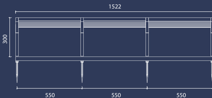
Frontansicht FLASH
