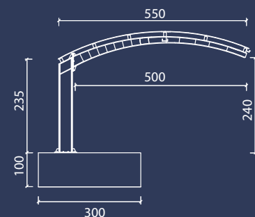
Seitenansicht SUNSHELL
