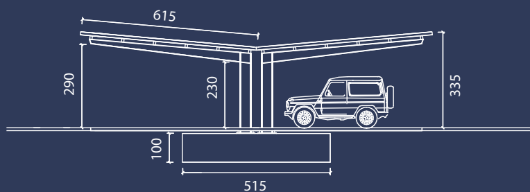
Seitenansicht ESPACE
