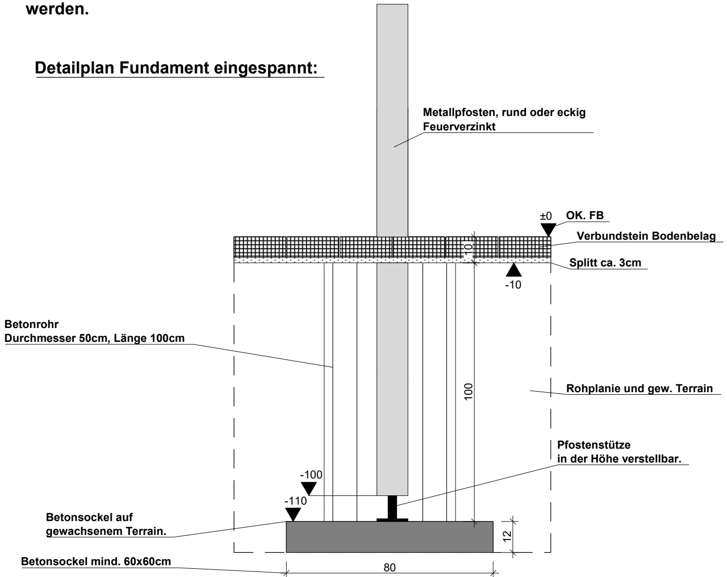
Bild eines Metallpfosten Eingespannt:
